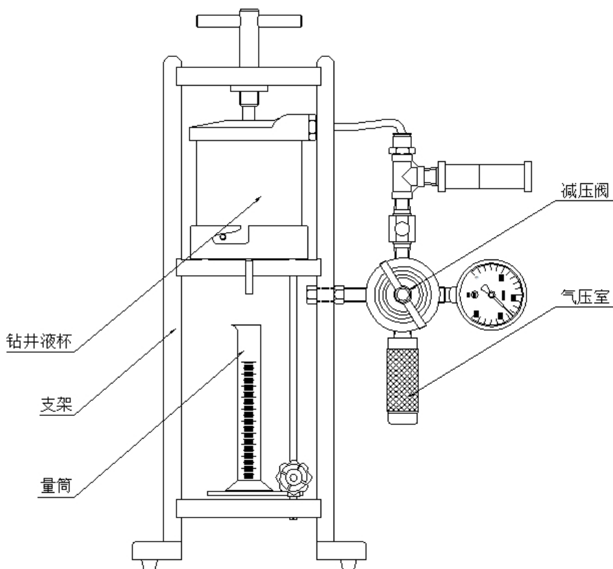
（图一）ZNS-5B 型中压滤失仪结构示意图
